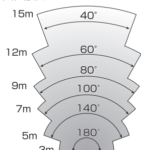
【平面図】検知エリアを上からみた図
