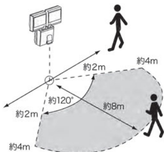
【平面図】検知エリアを上からみた図
