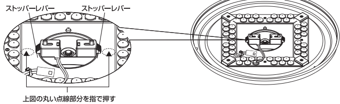
図2 アダプタユニットのストッパー部分 図3 本体を押し上げて取り付けた状態
