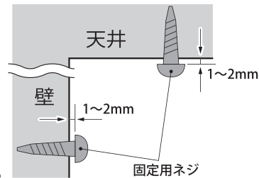
《取り付け寸法》
