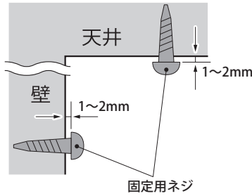
《取付寸法》
